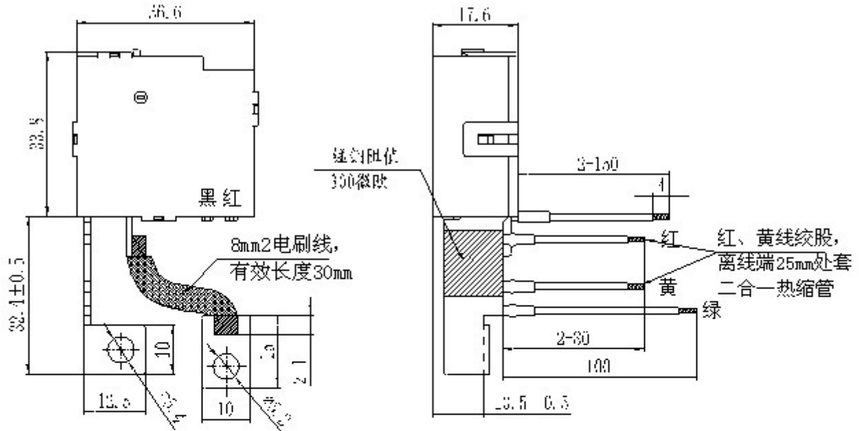
外形结构图 (单位: mm) Contour Chart (unit: mm)
