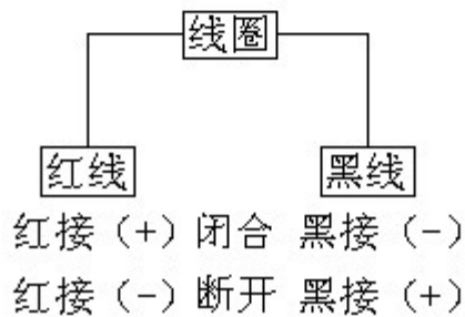
接线图
